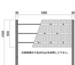
造作H900mm 参考寸法図
