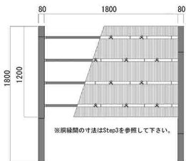
造作H1200mm 参考寸法図
