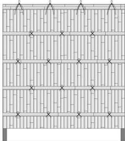
↓ 飾り縄 配置 参考図(造作H1800の場合)
