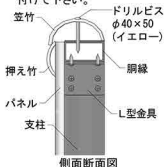
側面断面図
