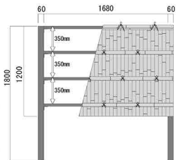
造作H1200mm 参考寸法図
