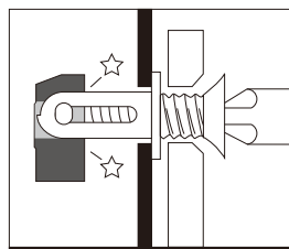
2. サラネジを一旦逆転→正転
