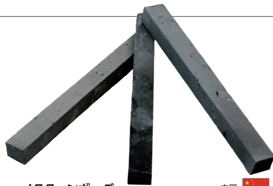
ノクターンボーダー 中国 商品コード サイズ(mm) 重量(kg) 設計価格/個 LBS-05B 約230×20×20 0.3 200円 使用数量/1㎡あたり 110個
