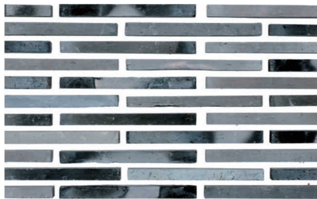
ノクターン 中国 商品コード サイズ(mm) 重量(kg) 設計価格/個 LBS-05 約230×50×20 0.6 250円 使用数量/1㎡あたり 65個
