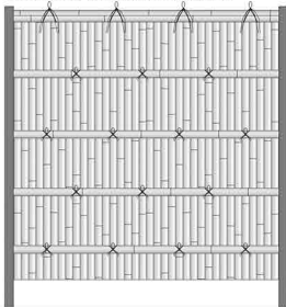
↓ 飾り縄 配置 参考図(造作H1800の場合)
