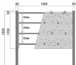
造作H1200mm 参考寸法図
