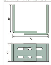
袖垣取付金具下部寸法図
