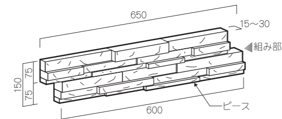
寸法図 (mm)
